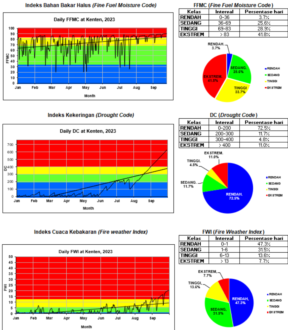
Gambar 26. Grafik FDRS Periode 1 Januari – 30 September 2023
